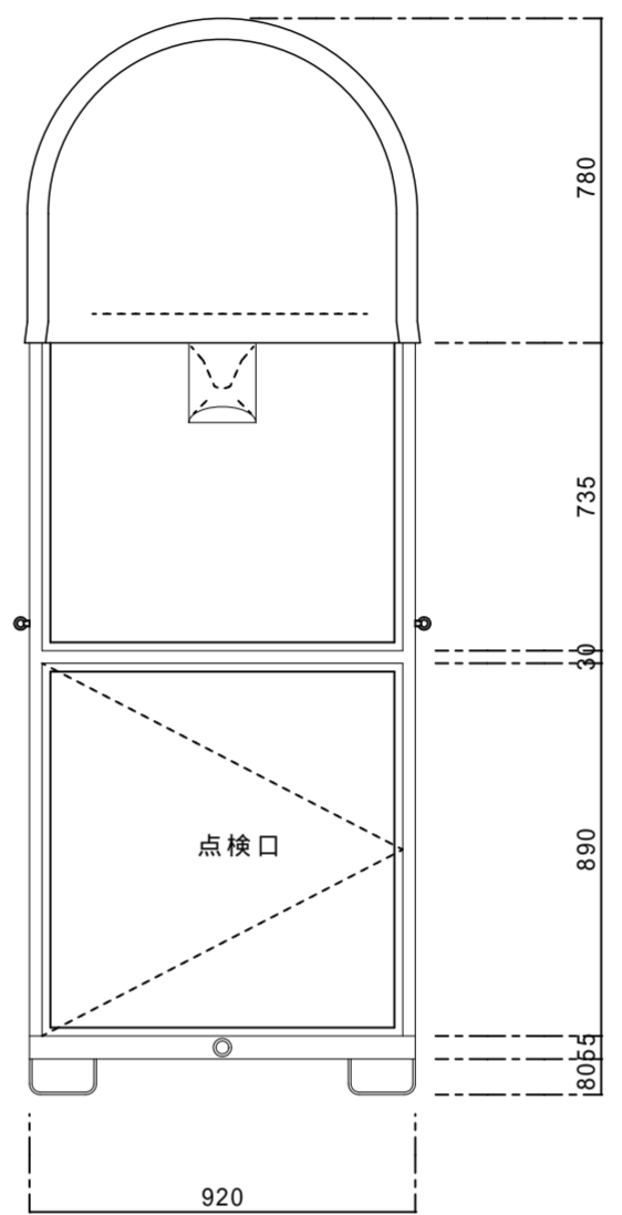
背面図
