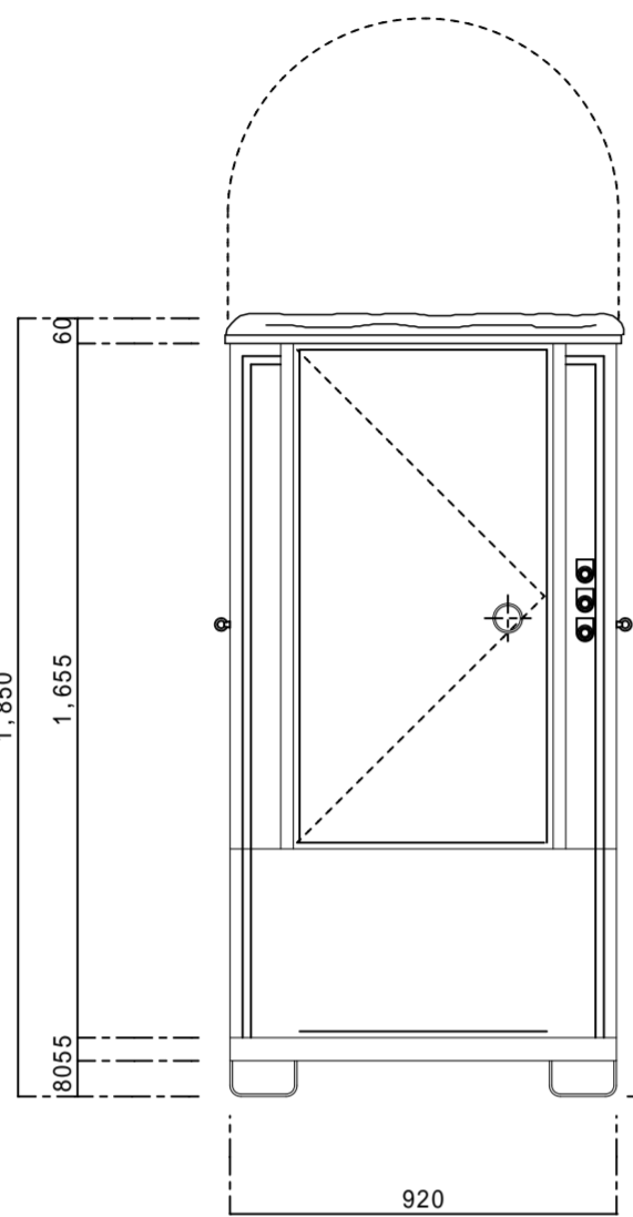
屋根折畳時
