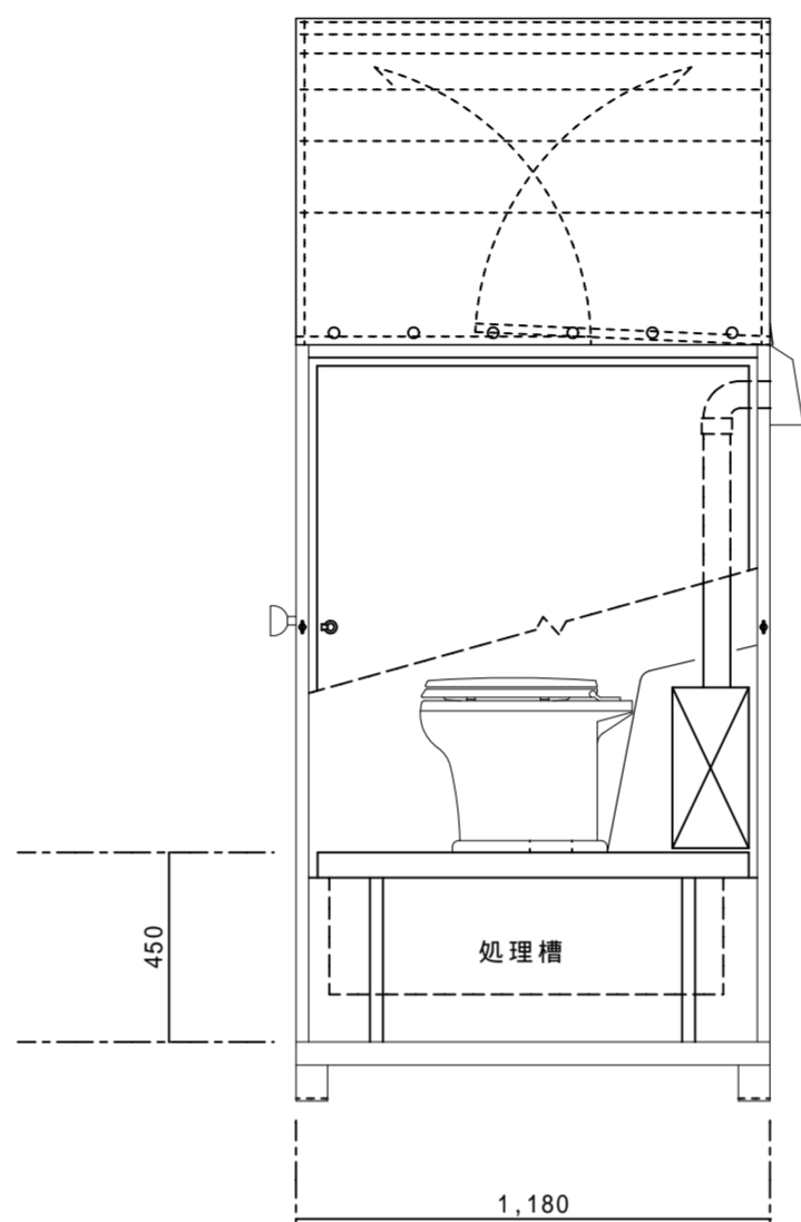
側面図
