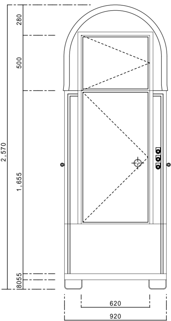
正面図
