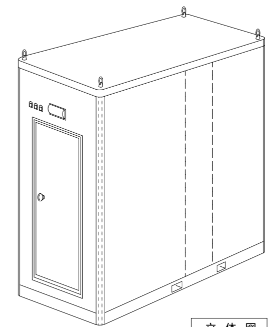
立体図
