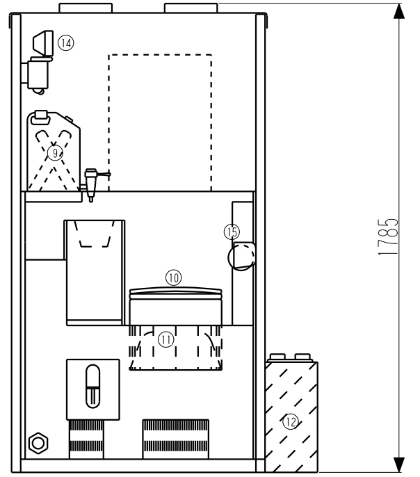
内観図
