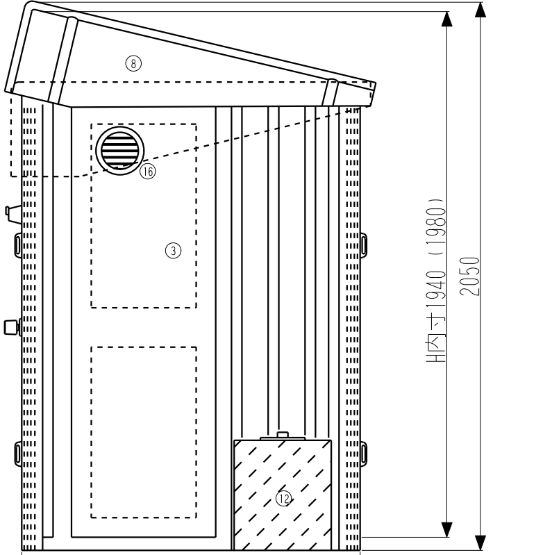
右側面図 (屋根組立時)
