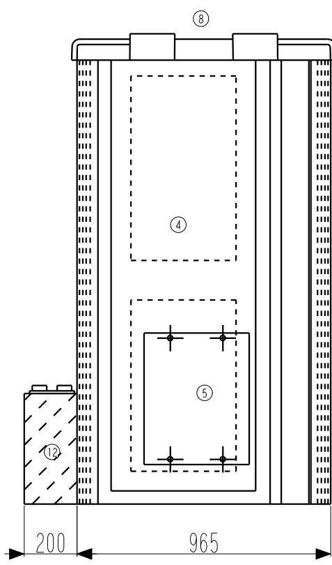
背面図 (屋根収納時)
