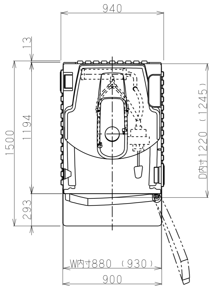
平面図
