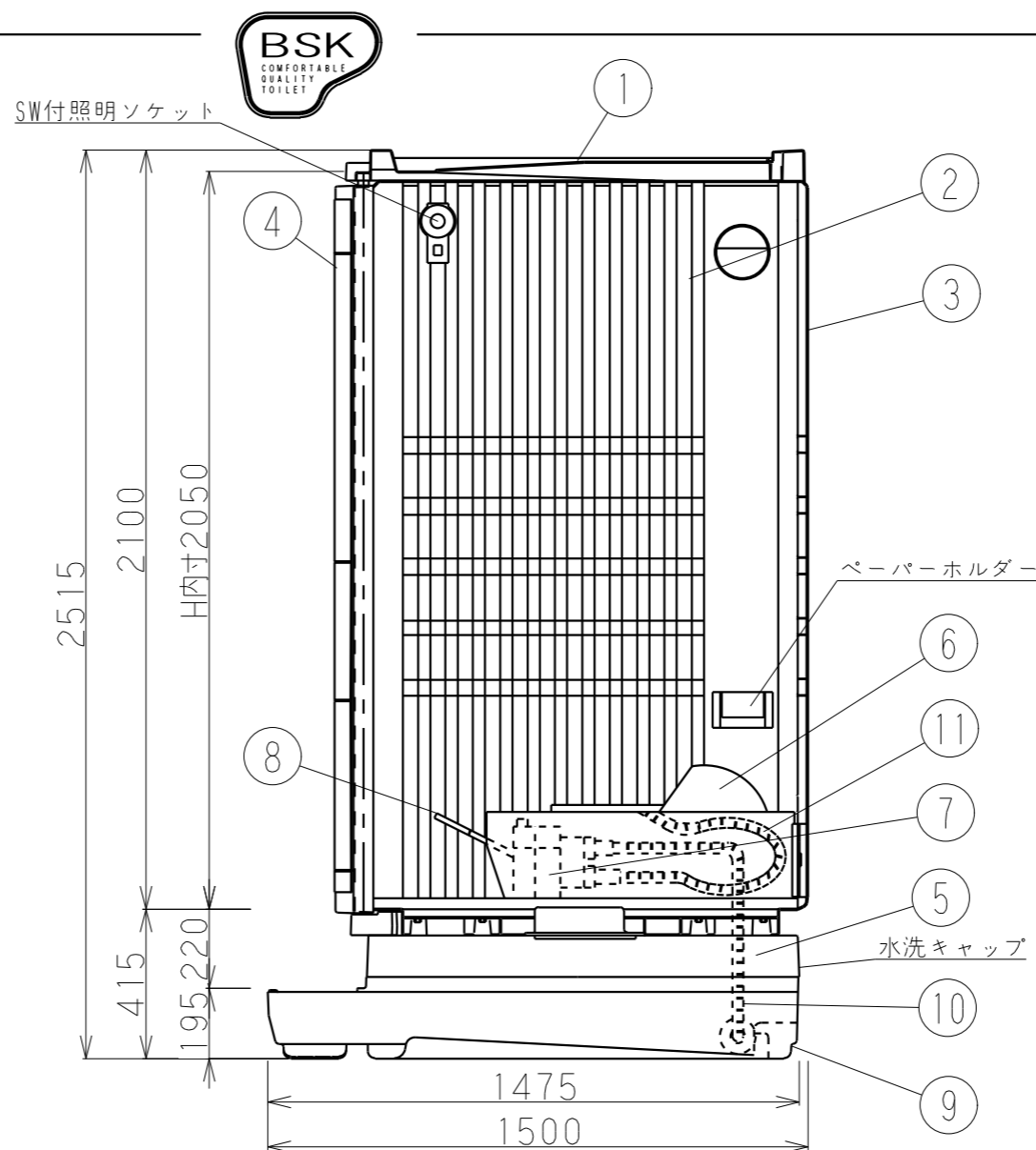
側面図
