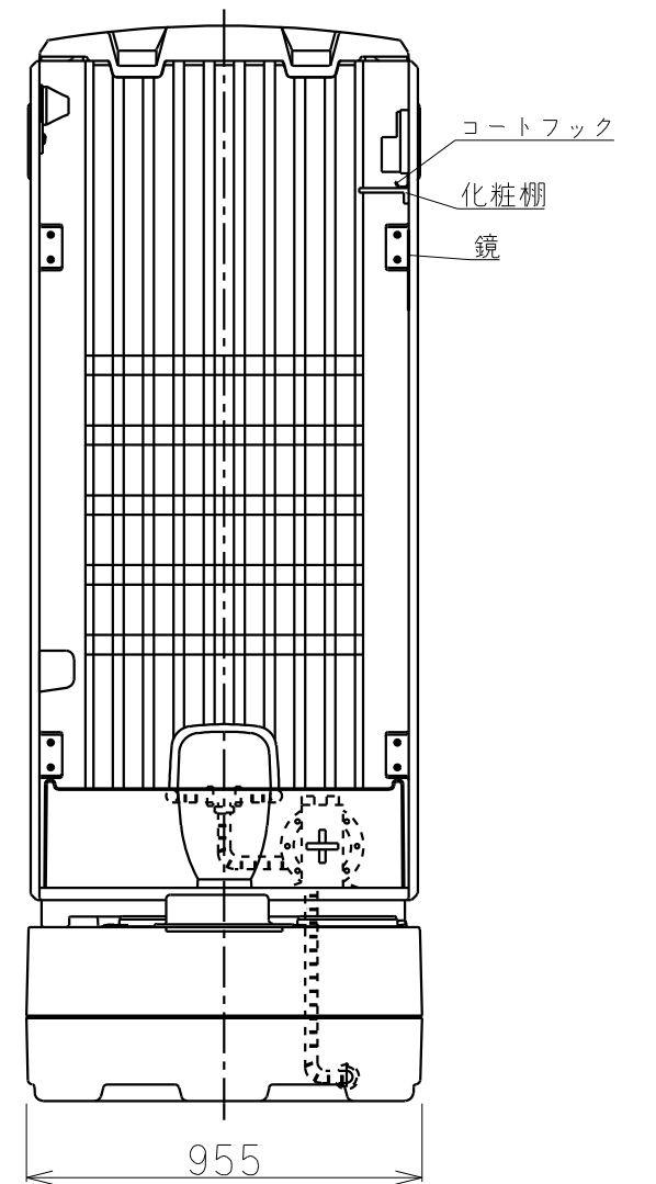
正面図
