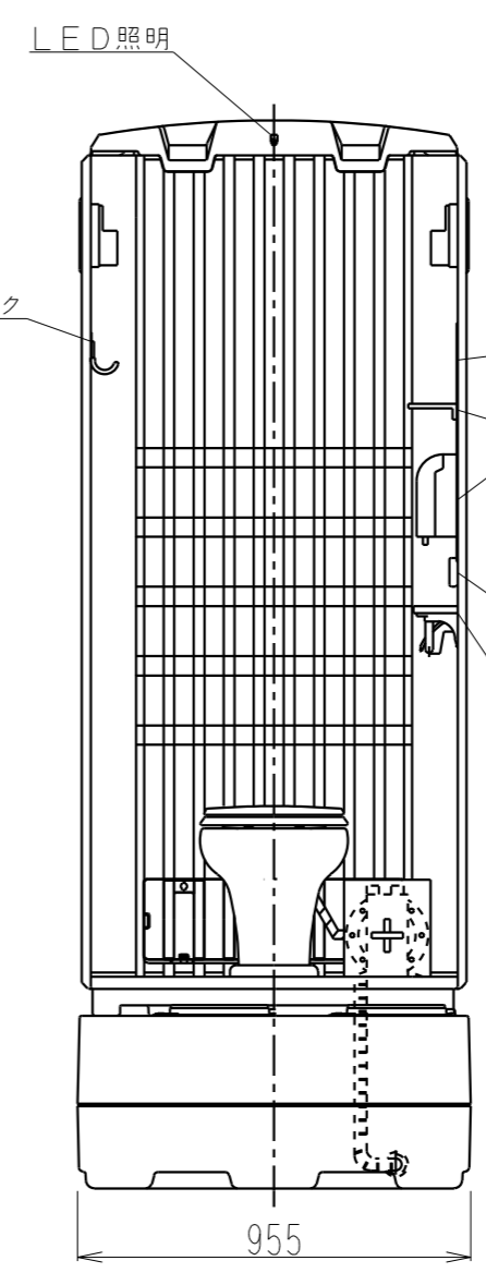
正面図
