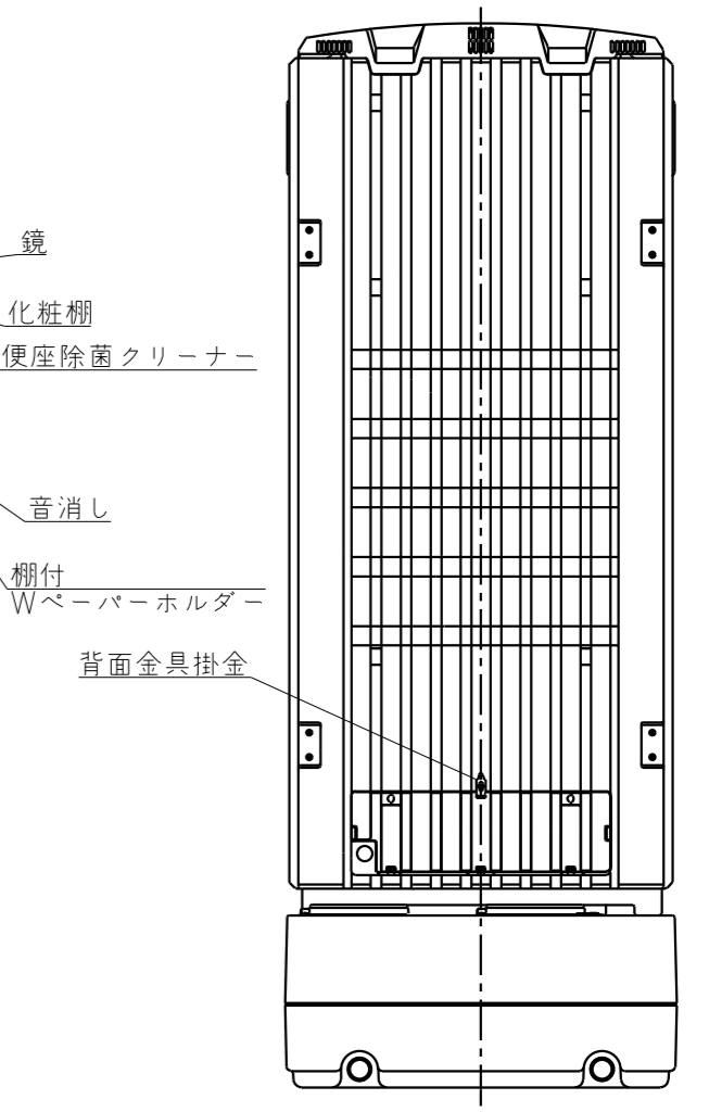
背面図
