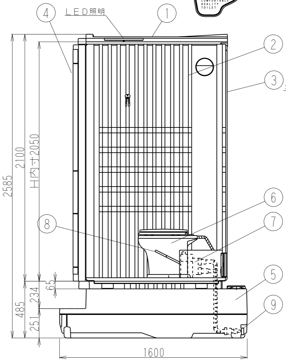
側面図
