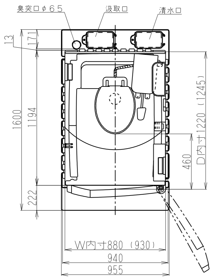
平面図
