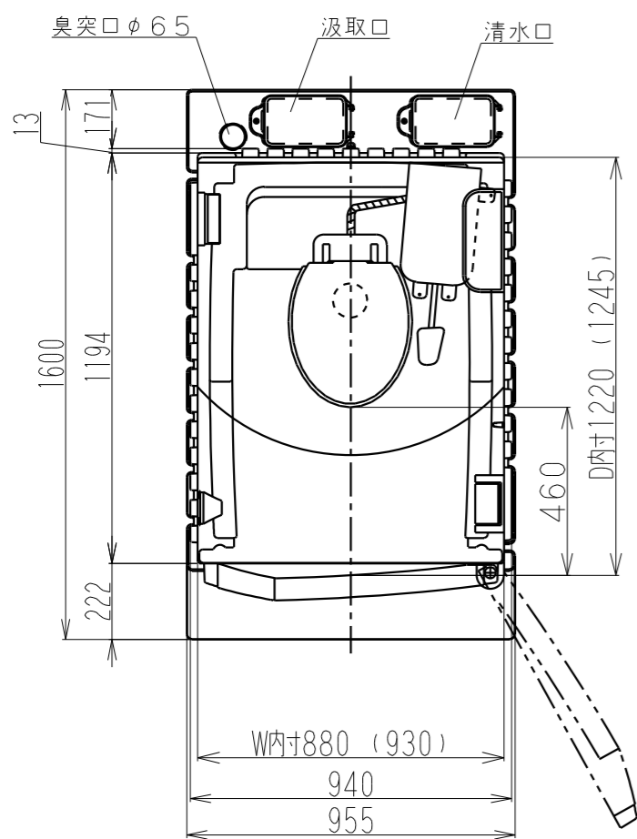
平面図
