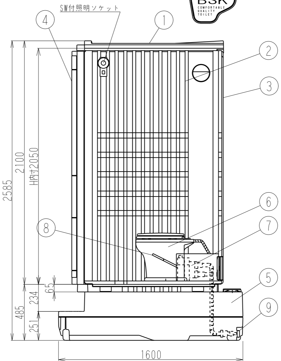
側面図
