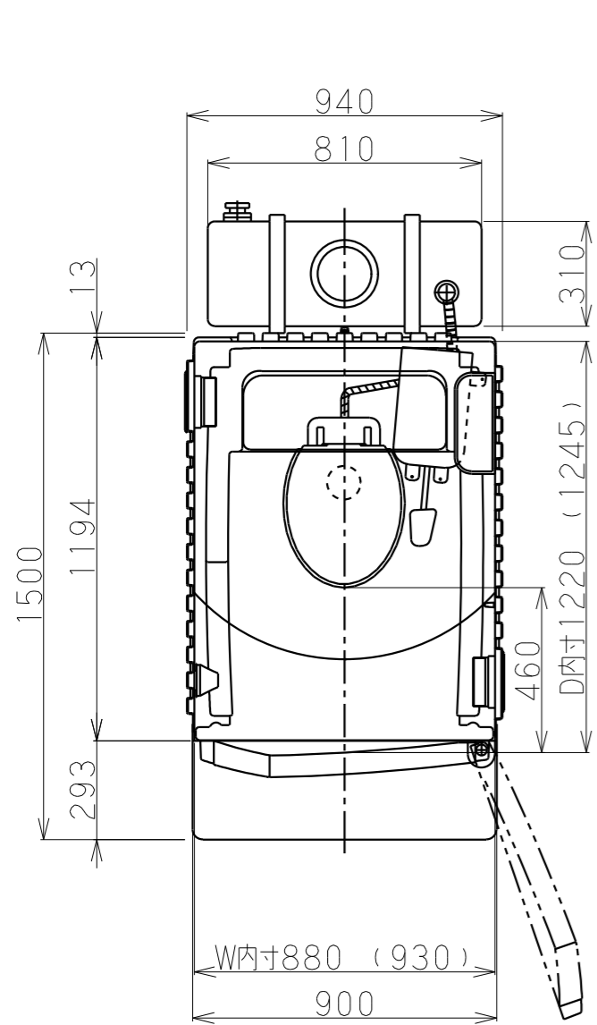
平面図
