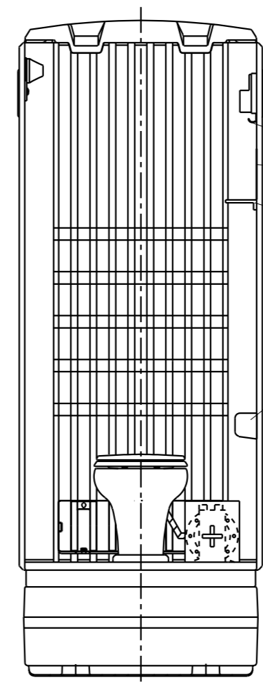
正面図
