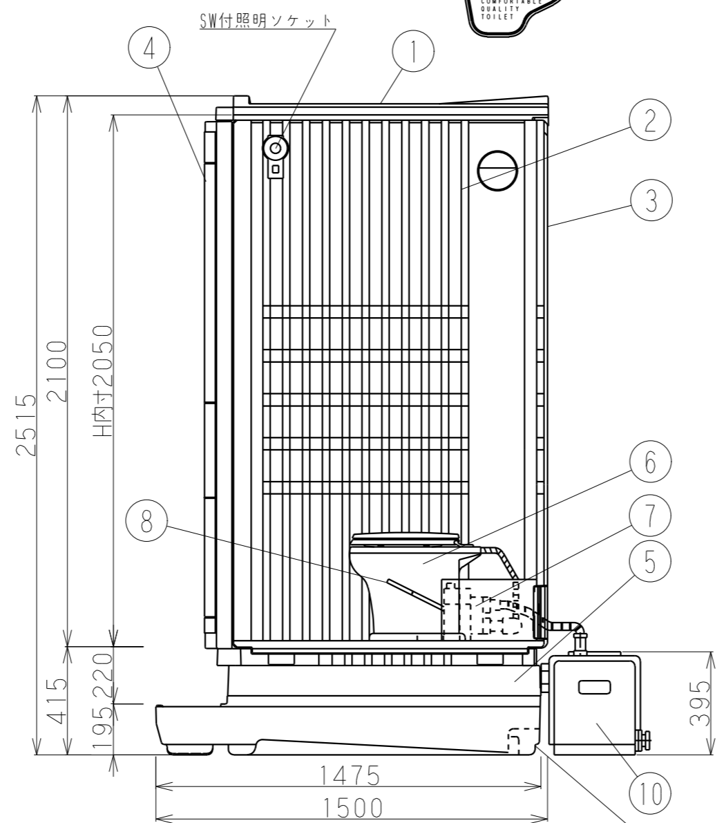
側面図
