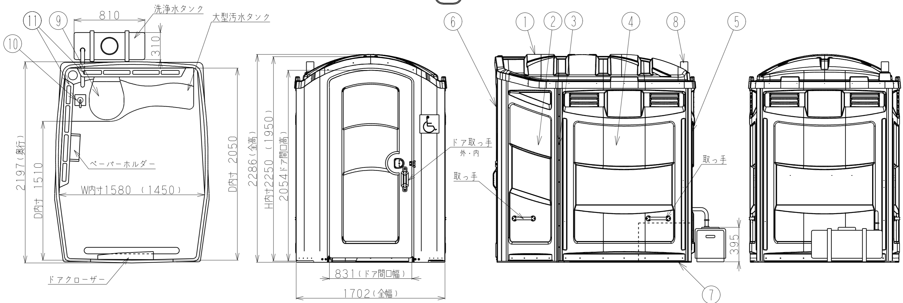
平面図
